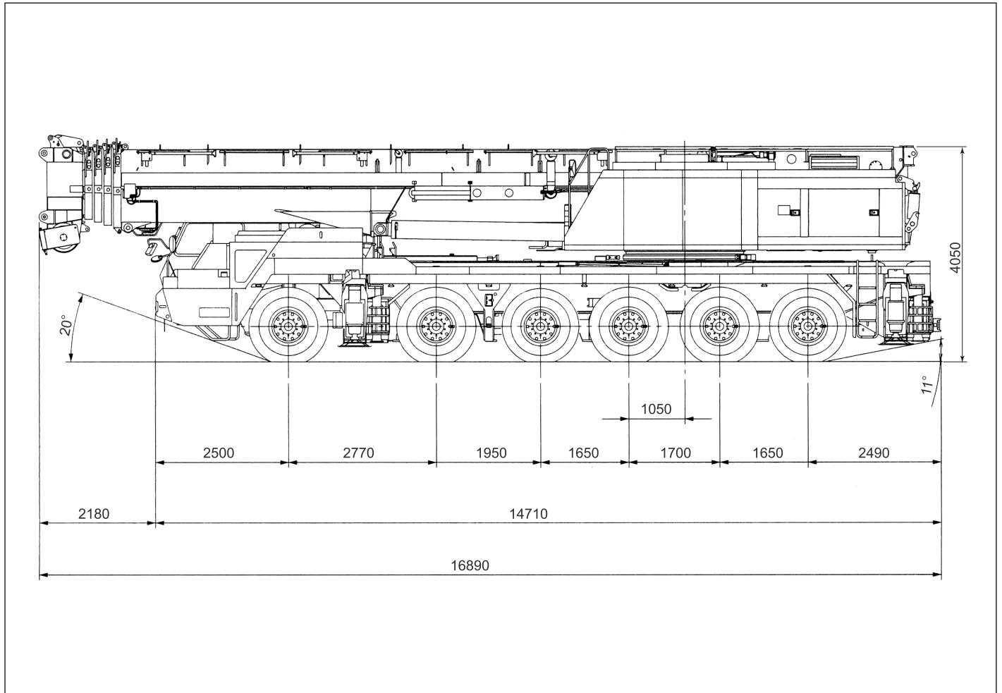
■クレーン用台車外観寸法
