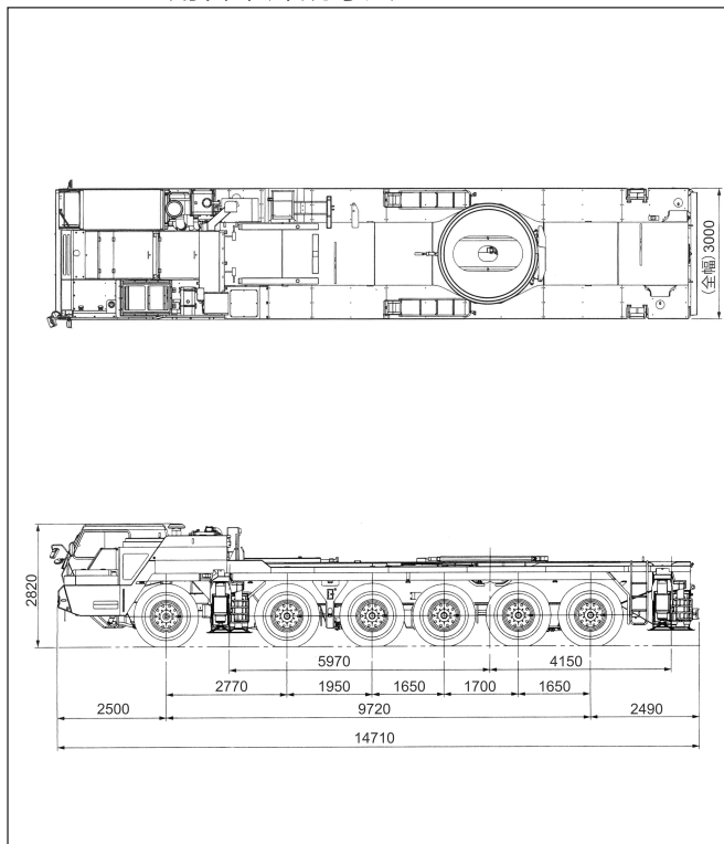
■クレーン用台車外観寸法
