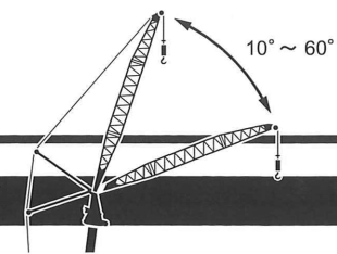
HA性能 40.9mブーム+4.4m+31.0mヘビーリフトジブ
